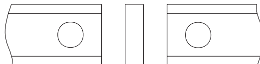
Lavorazioni: taglio e doppio foro Ø8
