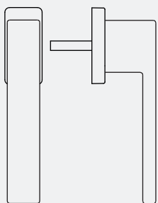
Martellina D.K. con movimento 4 scatti senza bussole con quadro 7
