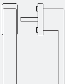
Martellina D.K. con movimento 8 scatti con bussole con quadro 7
