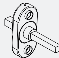
Movimento DK 8 scatti con bussole con quadro 7 (varie misure)
