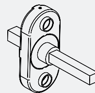
Movimento DK 4 scatti con bussole con quadro 7 (varie misure)
