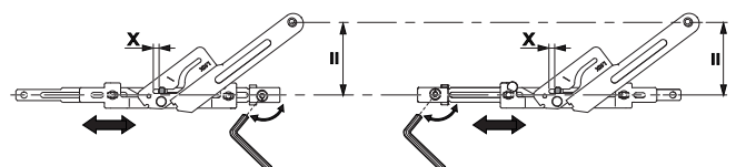
Parallelität Flügel-Rahmen durch Einstellung der Scheren
