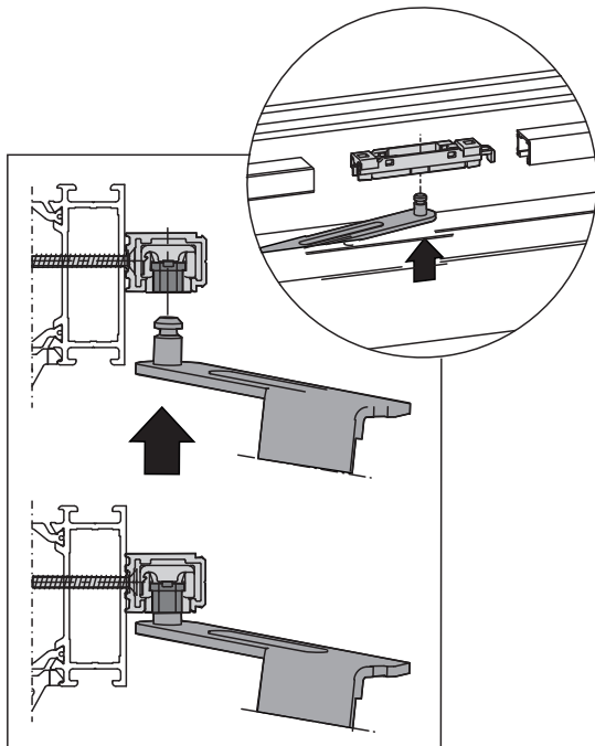
Scherenbefestigung
