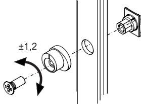
Einstellbarer Verriegelungs- bolzen
