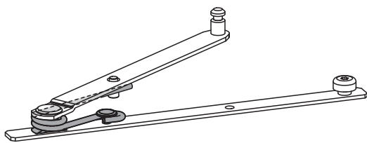
Zusatzschere
