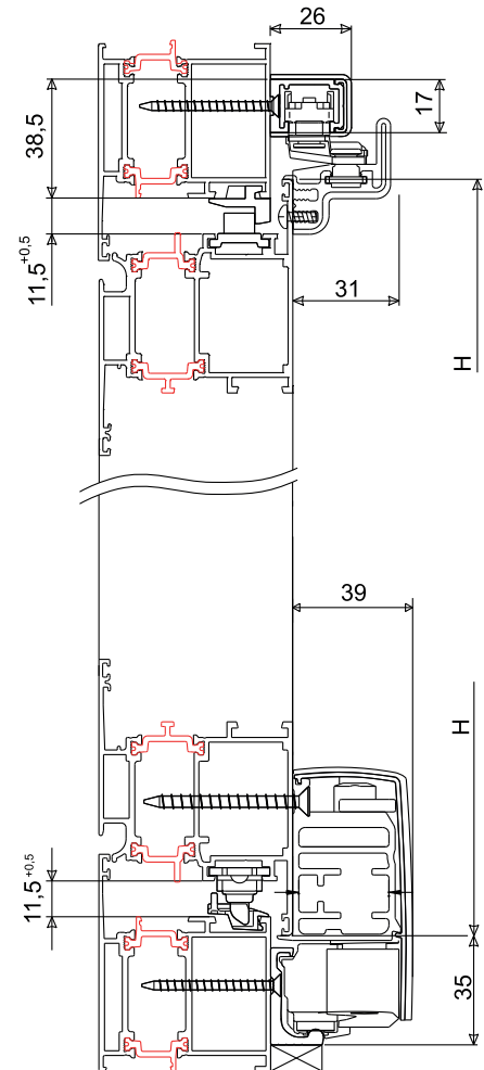
Sección aplicación
